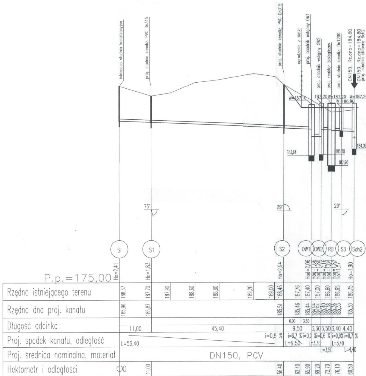
Profil podłużny ks na odc. Si-Sch2
